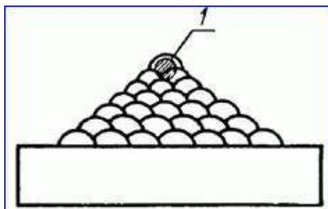
1-место отбора контрольных образцов
