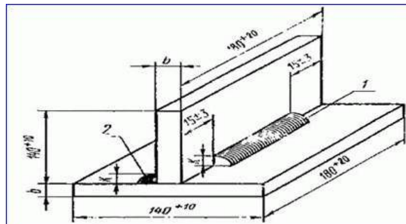
1 - контрольный сварной шов; 2 - сварной шов, обеспечивающий жесткость образца (выполняется только на двустороннем тавровом образце).
