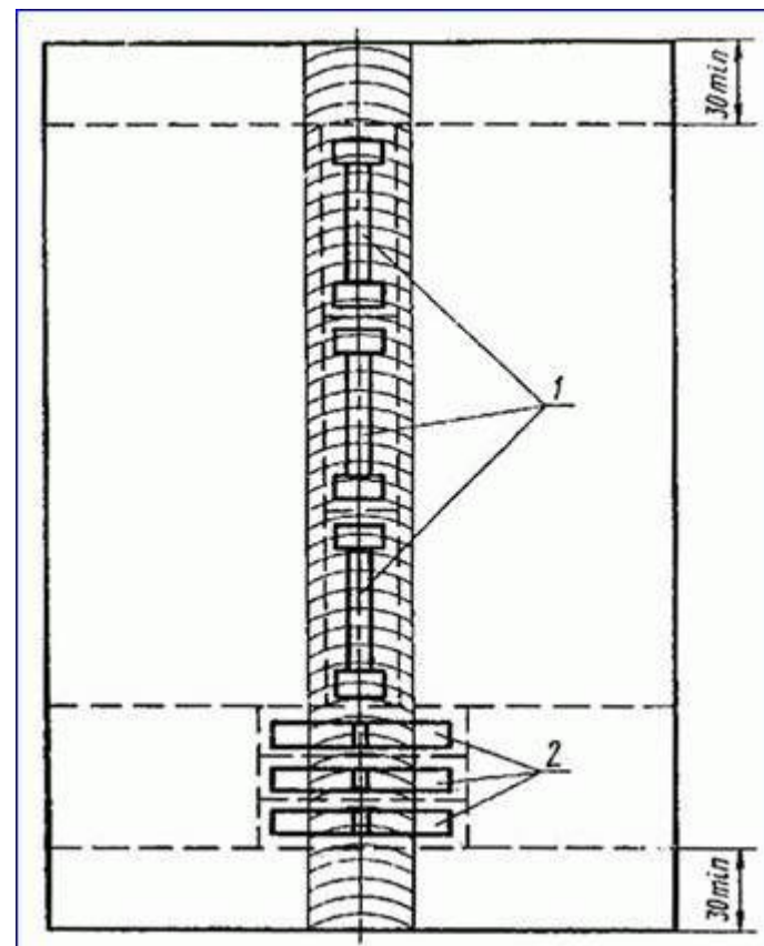
1 - образцы для испытания на статическое растяжение; 2 - образцы для испытания на ударный изгиб
